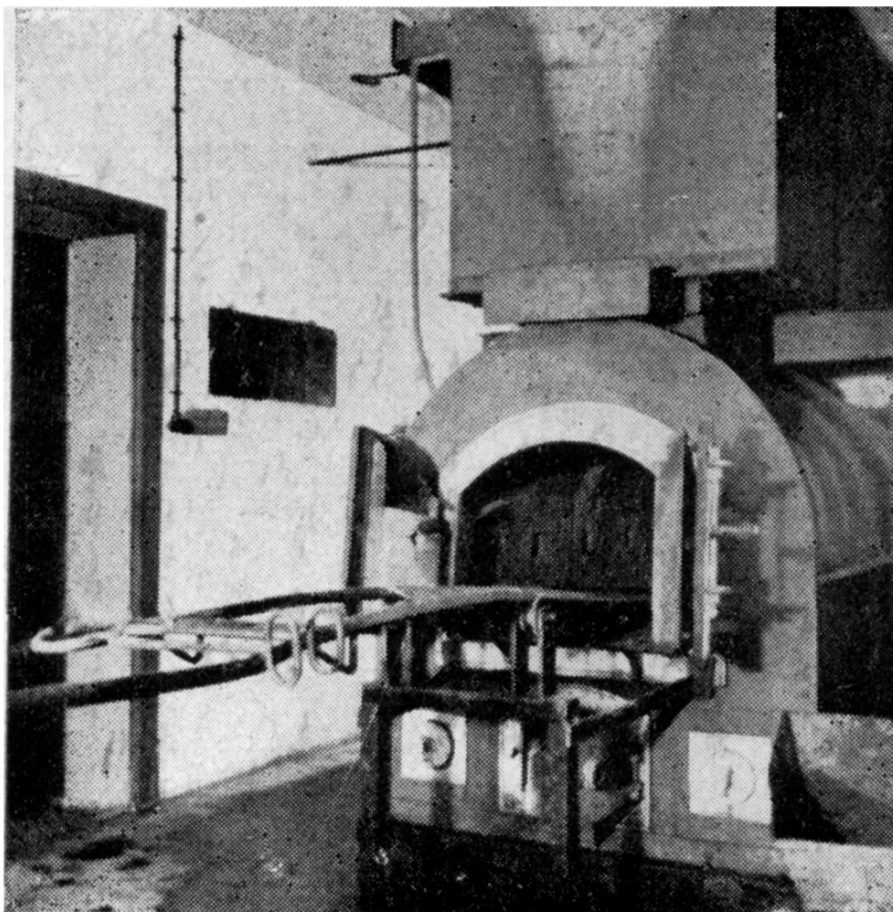
FOUR CRÉMATOIRE : gueulard ouvert
